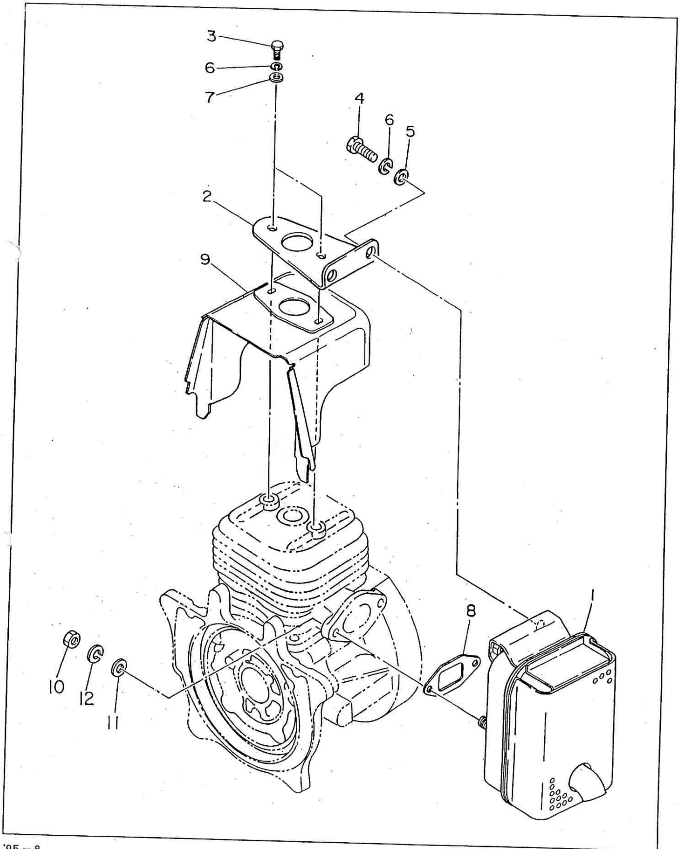
FIG. 3 MUFFLER
